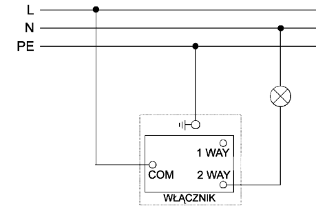
Schemat instalacji włącznika pojedynczego.
