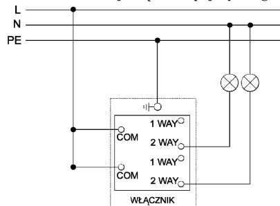
Schemat instalacji włącznika podwójnego.
