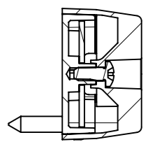
PRZEKRÓJ C-C
